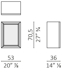
Vetrina Sopralzo chiusura con magnete / magnet closure
