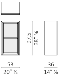
Vetrina Sopralzo chiusura con magnete / magnet closure
