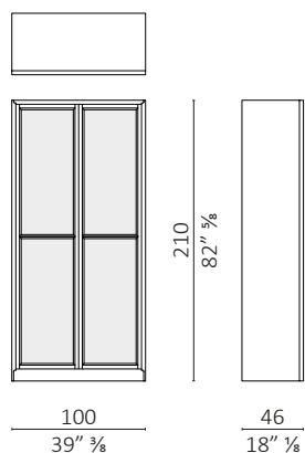
Vetrina chiusura con magnete/ magnet closure
