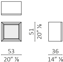
Vetrina Sopralzo chiusura con magnete / magnet closure
