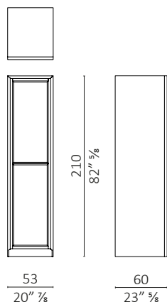
Armadio chiusura con magnete/magnet closure
