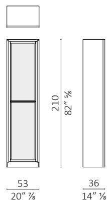
Vetrina chiusura cremonese/ cremone bolt closure
