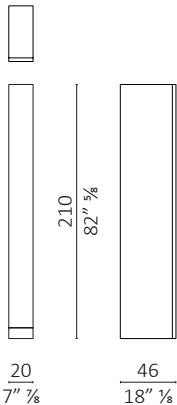
porta documenti/document holder
