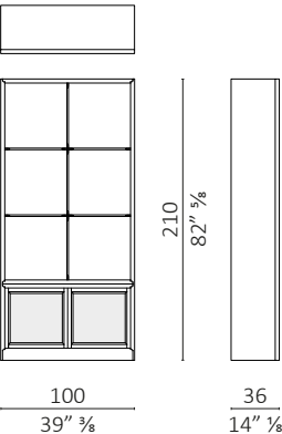
Libreria fissa con anta bassa/with low door
