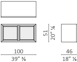
Vetrina Sopralzo chiusura con magnete / magnet closure
