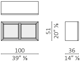
Vetrina Sopralzo chiusura con magnete / magnet closure
