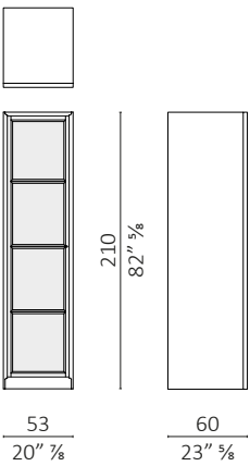
Armadio chiusura cremonese/cremone bolt closure
