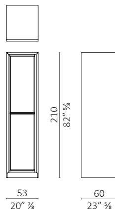
Armadio chiusura cremonese/cremone bolt closure
