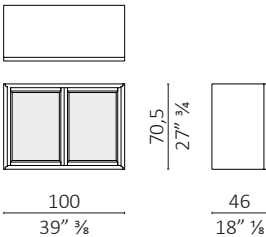
Vetrina Sopralzo chiusura con magnete / magnet closure
